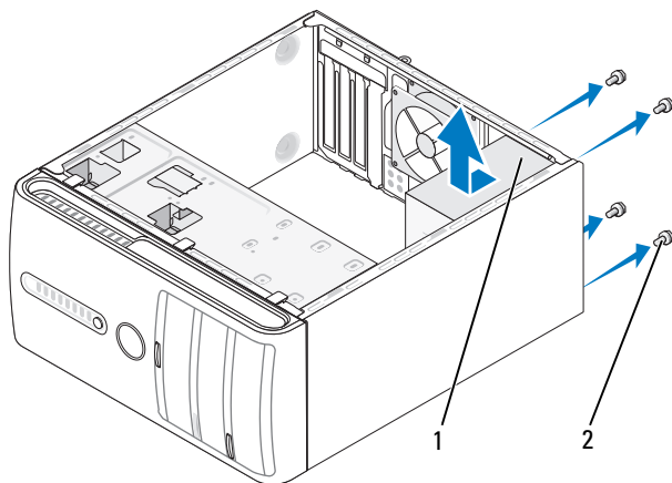
1 电源设备
